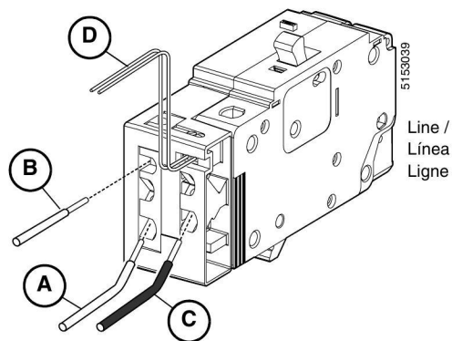
FIG. 2 : Wiring / Alambardo / Câblage
